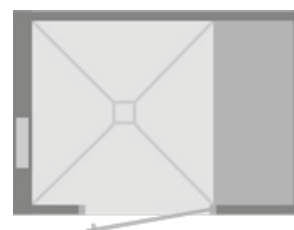
CAB-R 1780/1250 R.RL * Tür DIN rechts / Sitzbank rechts der Tür / Installationswand links der Tür
