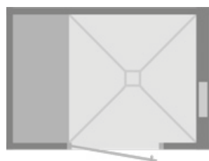
CAB-R 1780/1250 L.LR * Tür DIN links / Sitzbank links der Tür / Installationswand rechts der Tür
